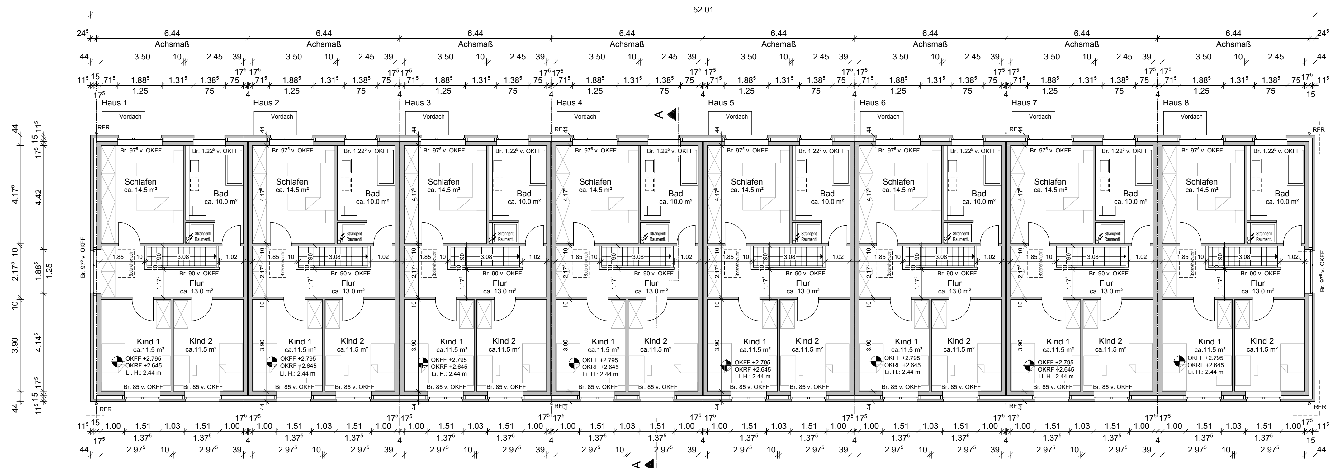
GRUNDRISS OBERGESCHOSS
