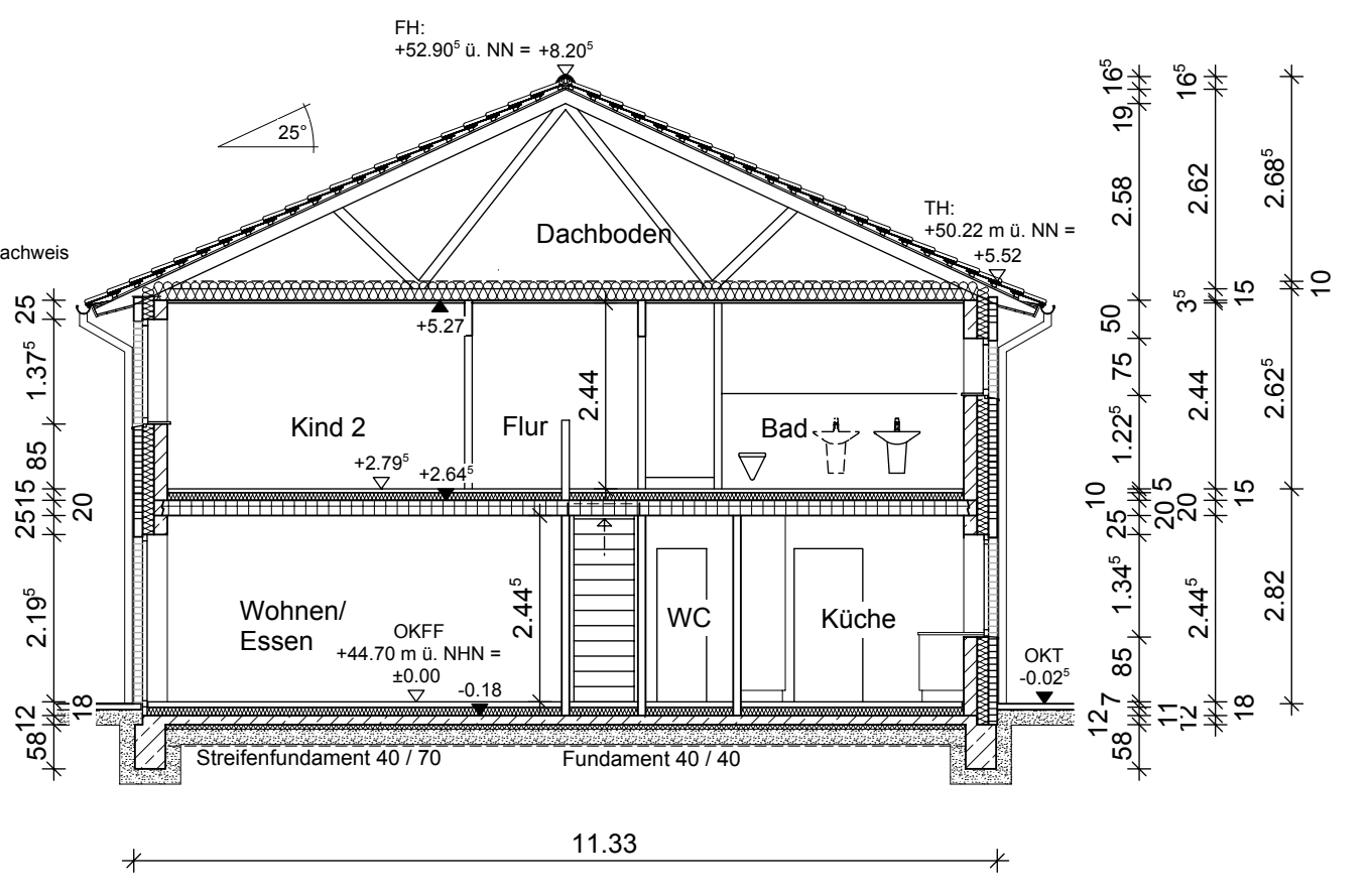
SCHNITT
