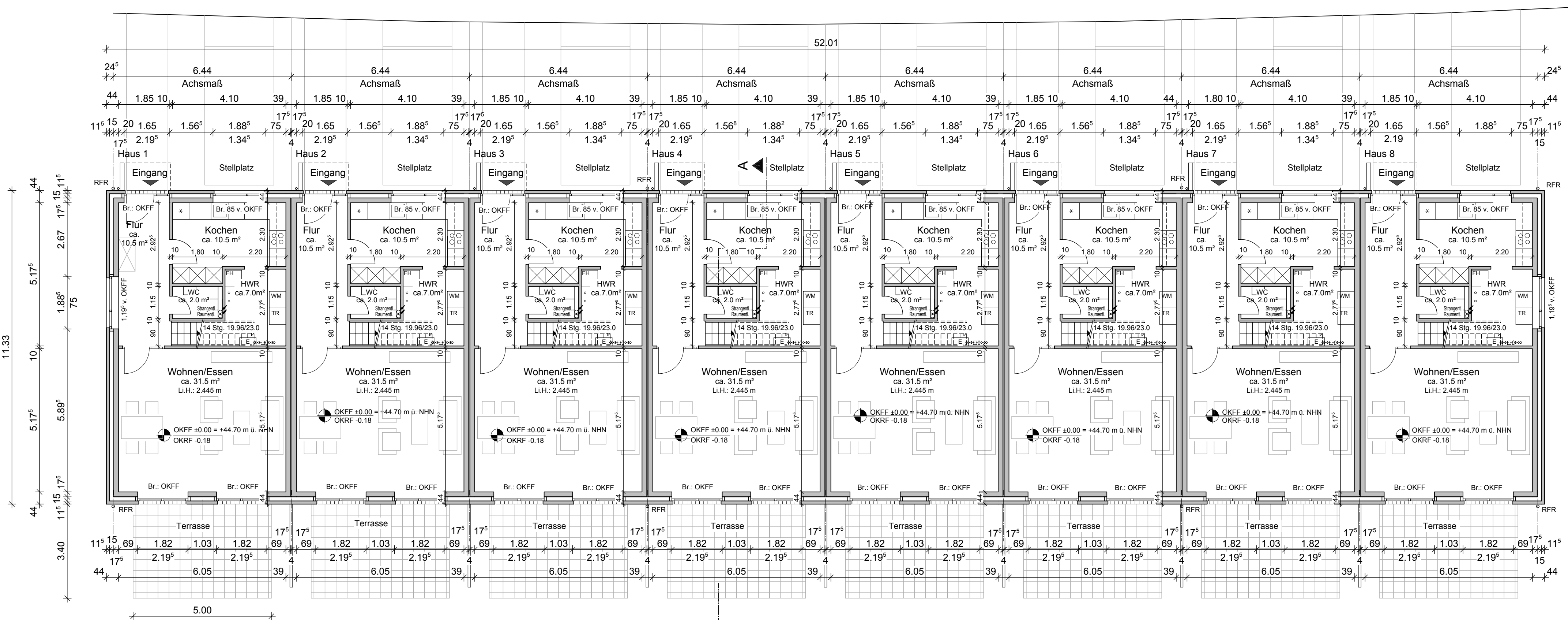
GRUNDRISS ERDGESCHOSS
